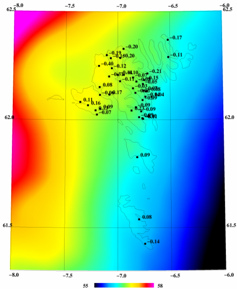
Fig. 7. Forskelle mellem N^{GPS} i gamle system og den nye gravimetrisk geoide.
