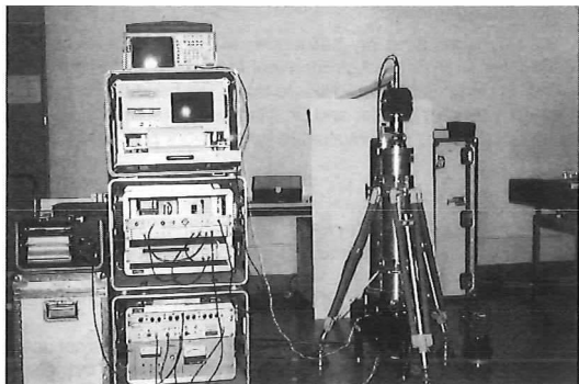
Fig. 1: The absolute gravimeter JILAG-6
